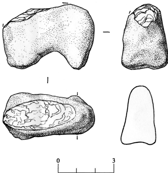
Рис. 3. Поселение Ракушечный Яр. Раскопки 2016 г. Керамическая зооморфная статуэтка.
