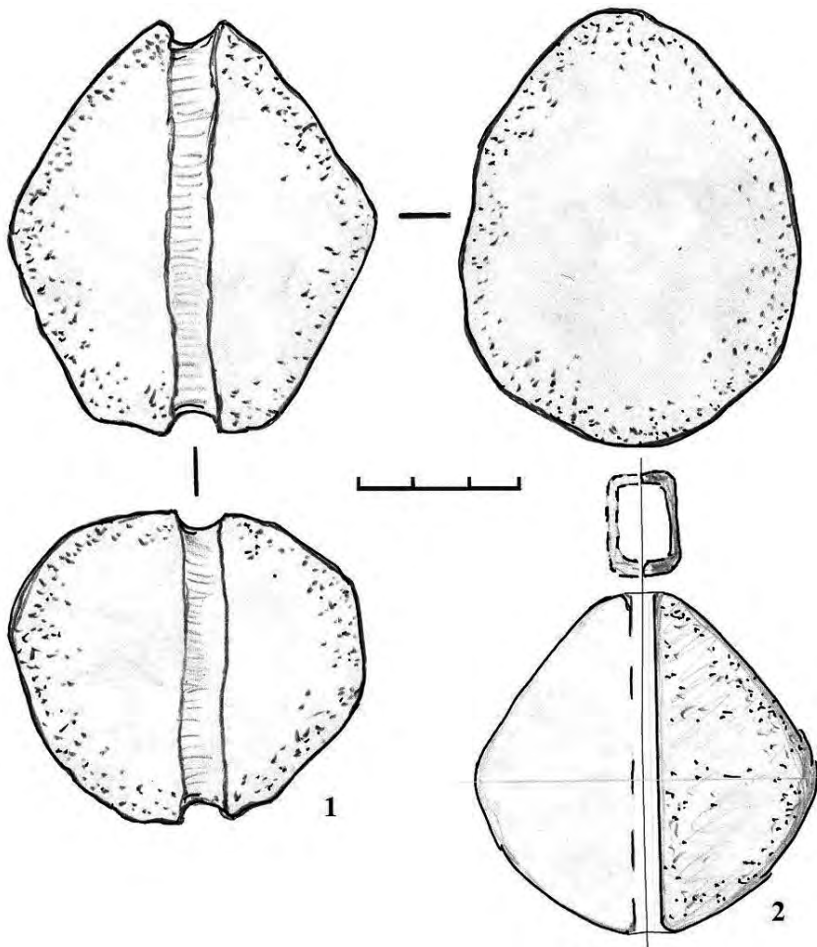
Рис. 3. Ударные части кистеней. Камень
